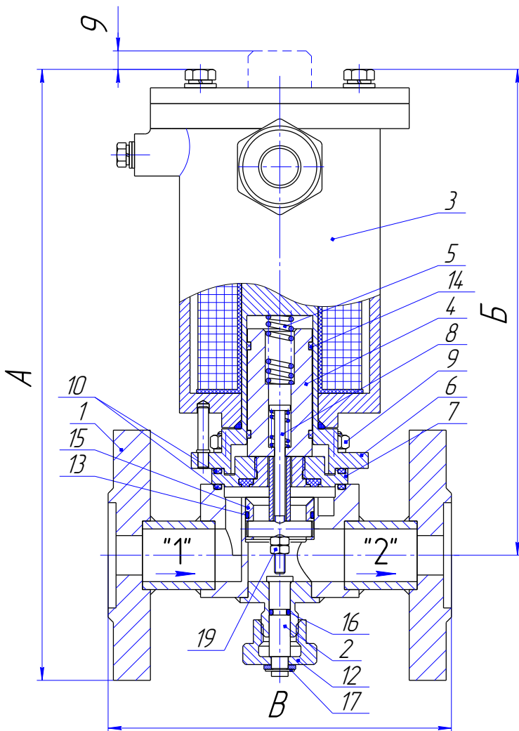
Рис. 1а. Клапан фланцевый. Общий вид.
