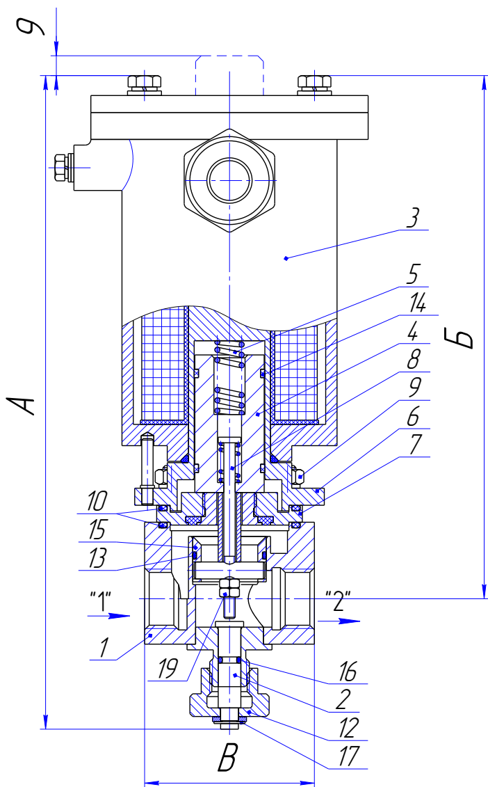
Рис. 16. Клапан муфтовый. Общий вид.
